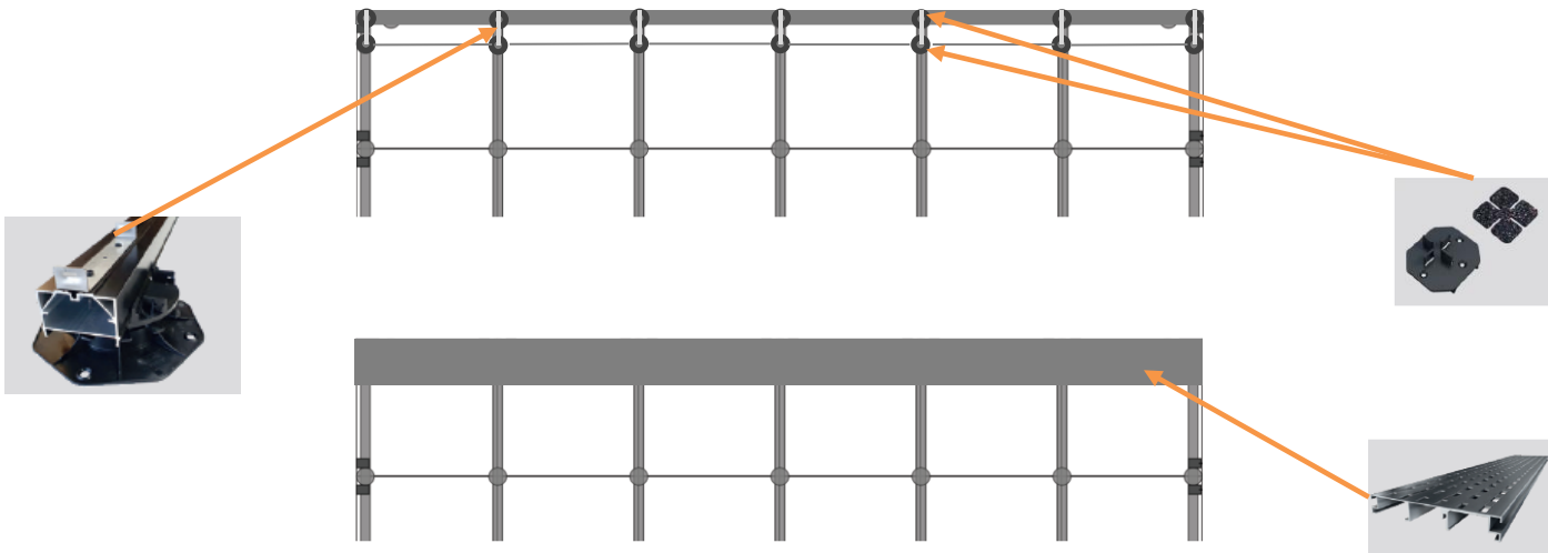
Drainage- und Belüftungsprofil Montageklammer
