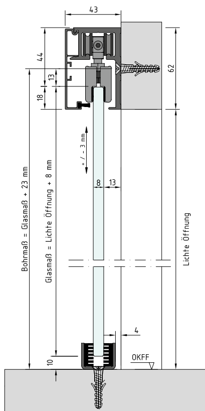
Montage mit Ganzglastür
