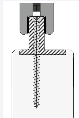
L&H T-Profil eingelassen und verschraubt
