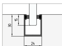
Seiten- und Oberlichthalter Oberfläche: Edelstahl matt
