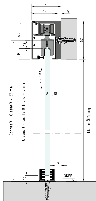
Montage mit Ganzglastür und 5 mm Hinterfüterung zur Erhöhung des Wandabstandes von 13 mm auf 18 mm, z. B. bei breiteren Sockelleisten
