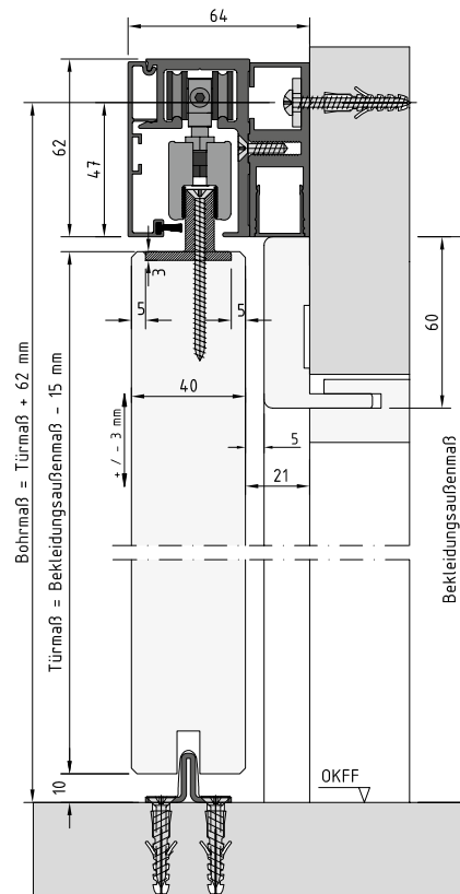
Montage mit Holztür
